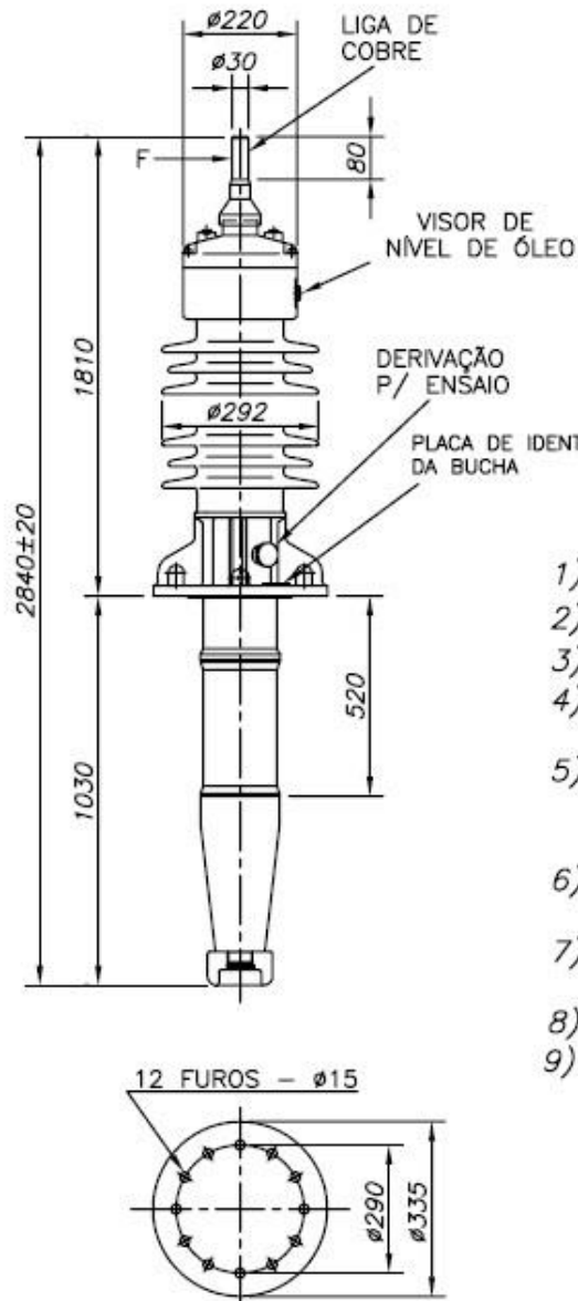
FIGURA 1 - CARACTERÍSTICAS GERAIS TB-BC 145 TOSHIBA
